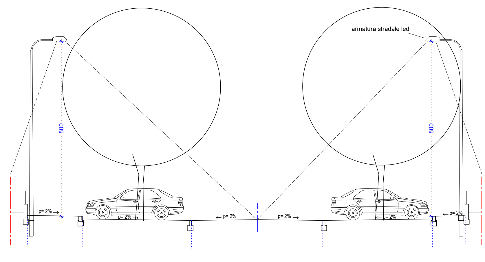
SEZIONE 3 - 3'
