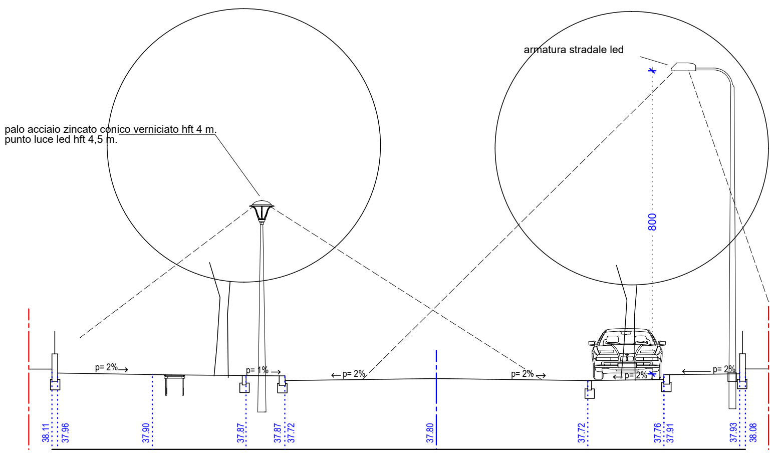
SEZIONE 2 - 2'
