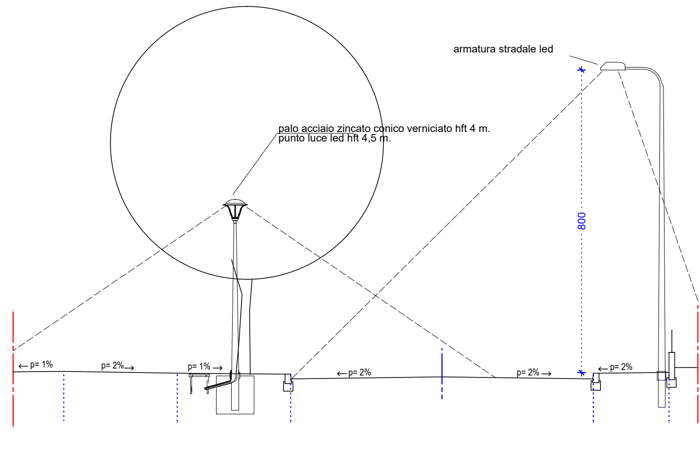
SEZIONE 5 - 5'
