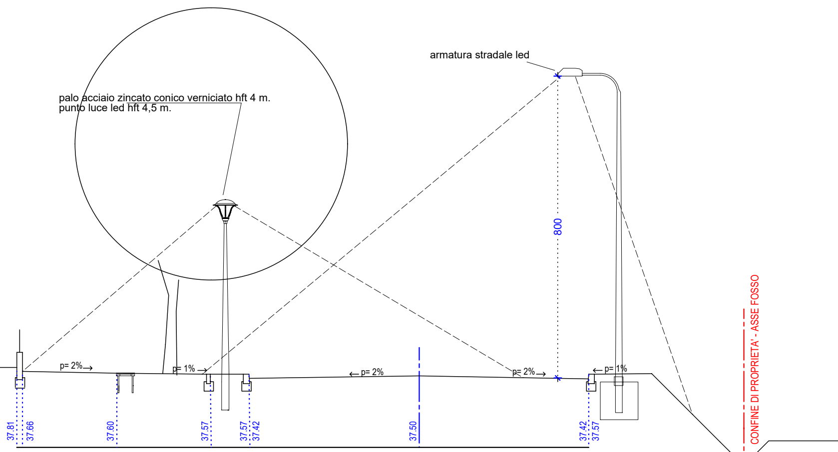
SEZIONE 1 - 1'
