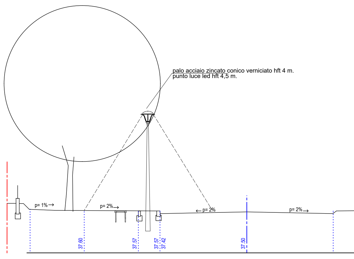
SEZIONE 7 - 7'
