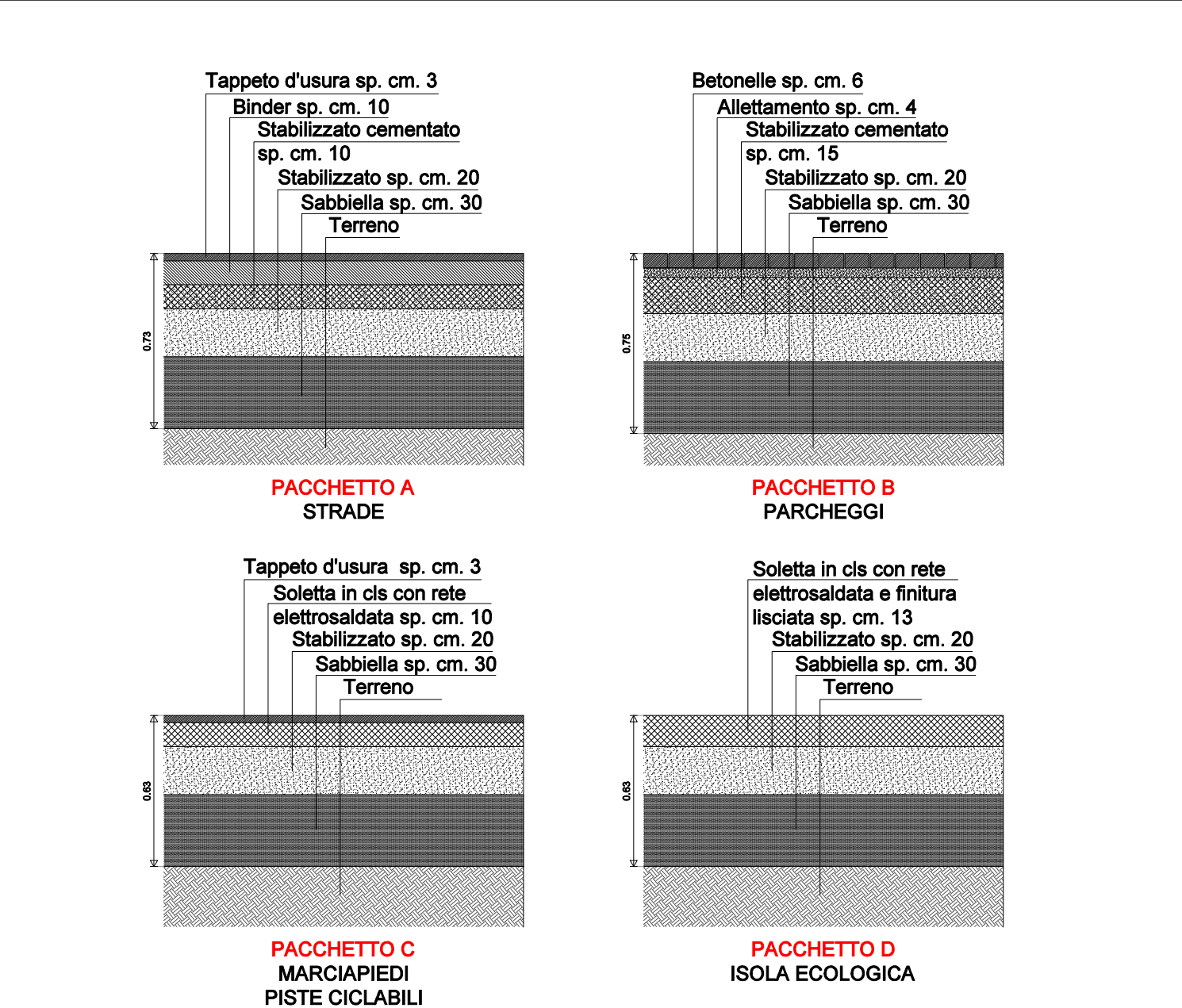
Stratigrafie tipo _ scala 1:25
