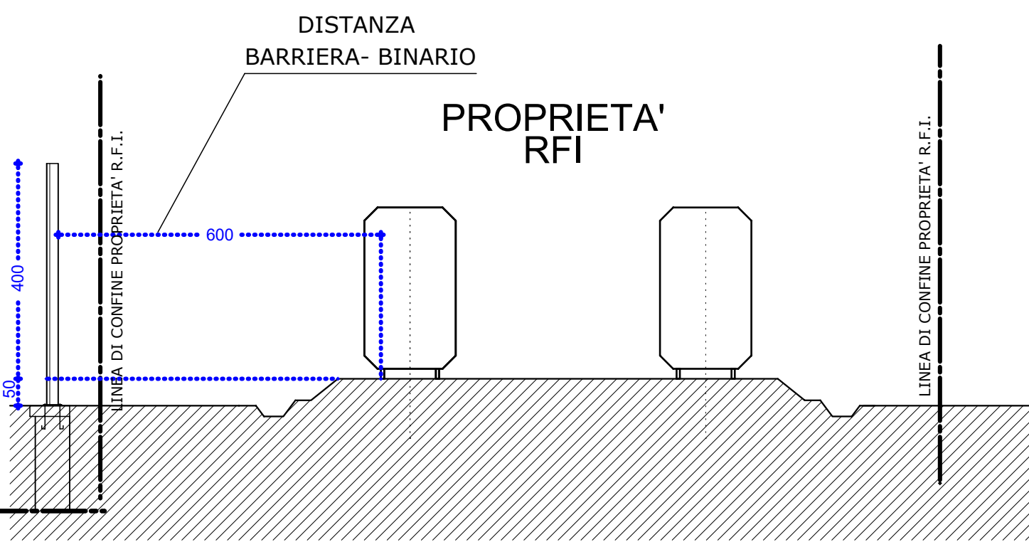
SEZIONE TRASVERSALE BINARI XX - scala 1:100
