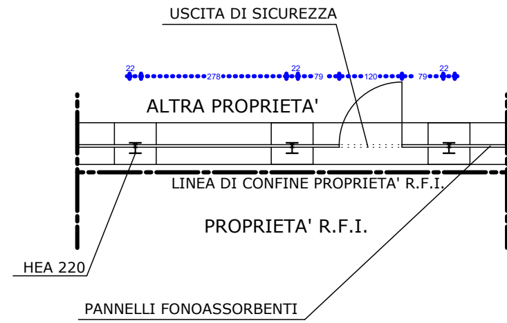
PARTICOLARE PIANTA - scala 1:50
