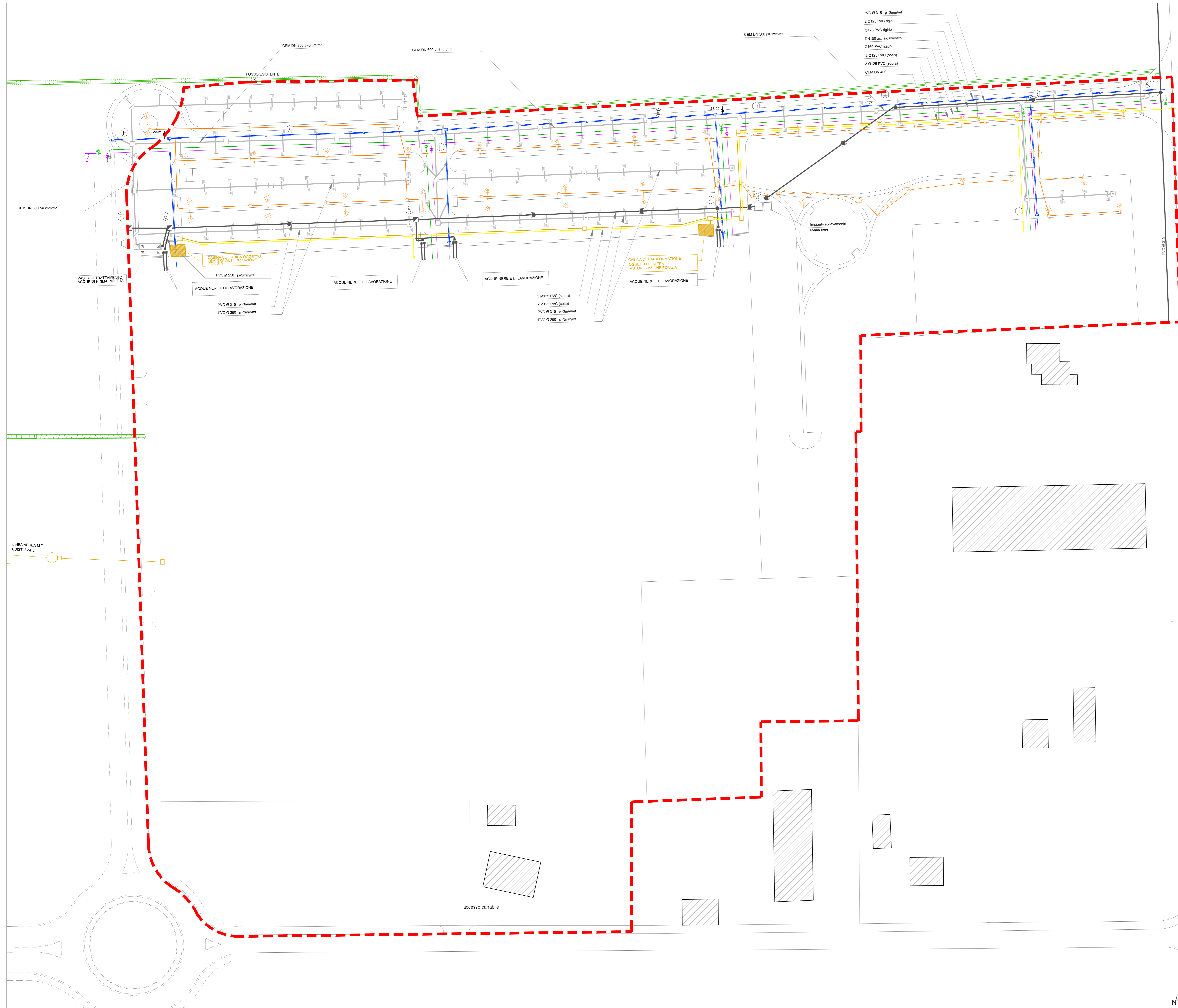
Rilievo planimetrico reti infrastrutturali esistenti 1: 500
